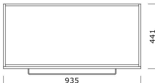
テレビ台用
