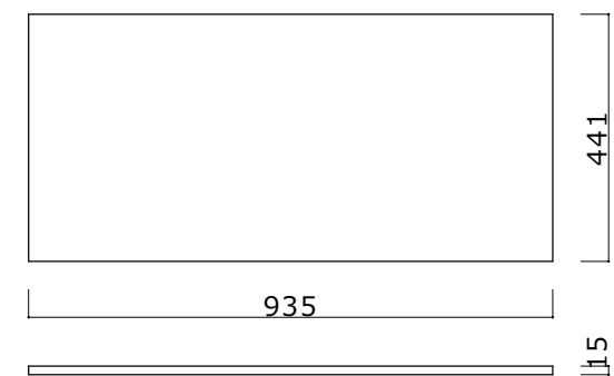
棚板 2段用
